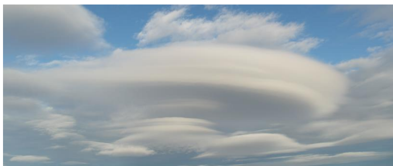
Skyformasjon over Hopen 27.05.13. En typisk midlere 4 – Altopcumulus lenticularis.
